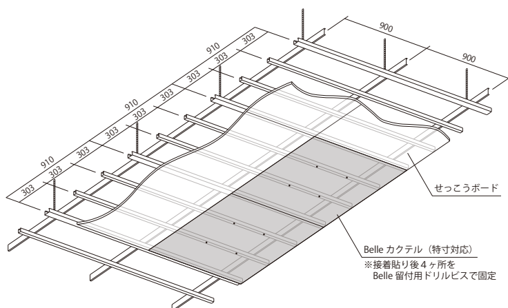
Belle カクテル天井施工図
