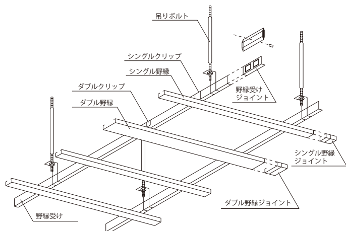
鋼製下地図
