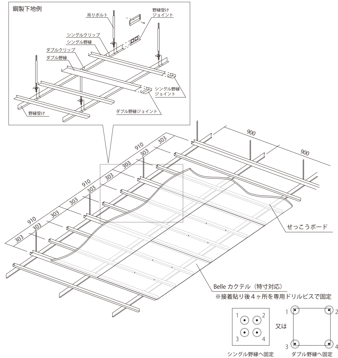
図3 Belleカクテル 天井施工図
